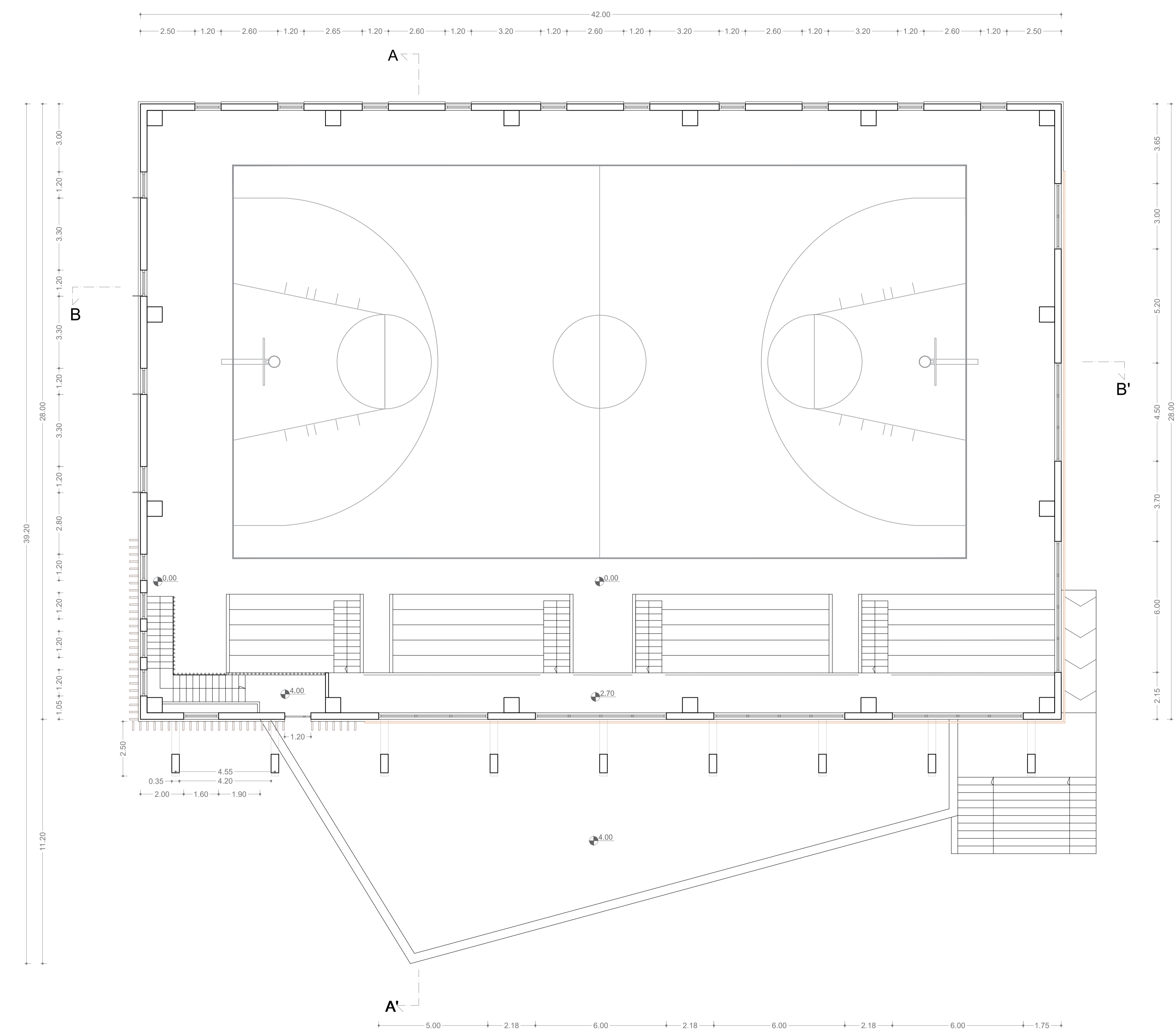
PIANTA QUOTA + 5.00
