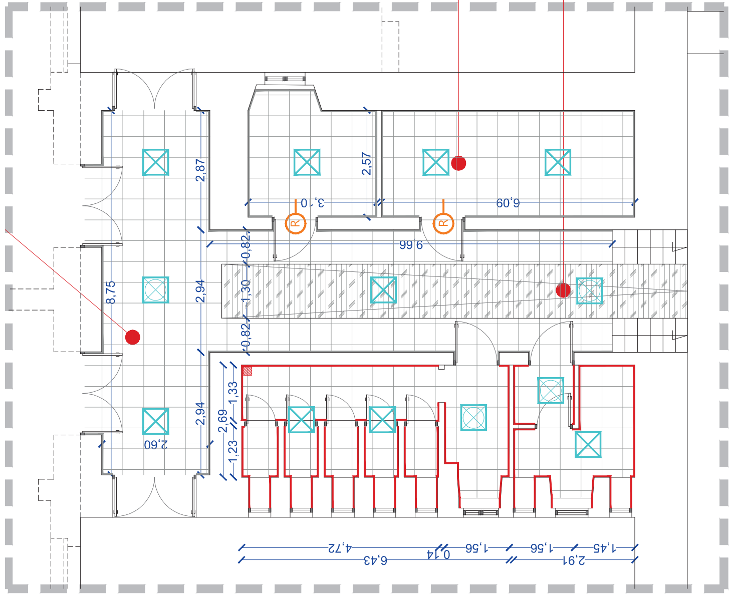
STRALCIO PIANTA DEL PIANO INTERRATO
