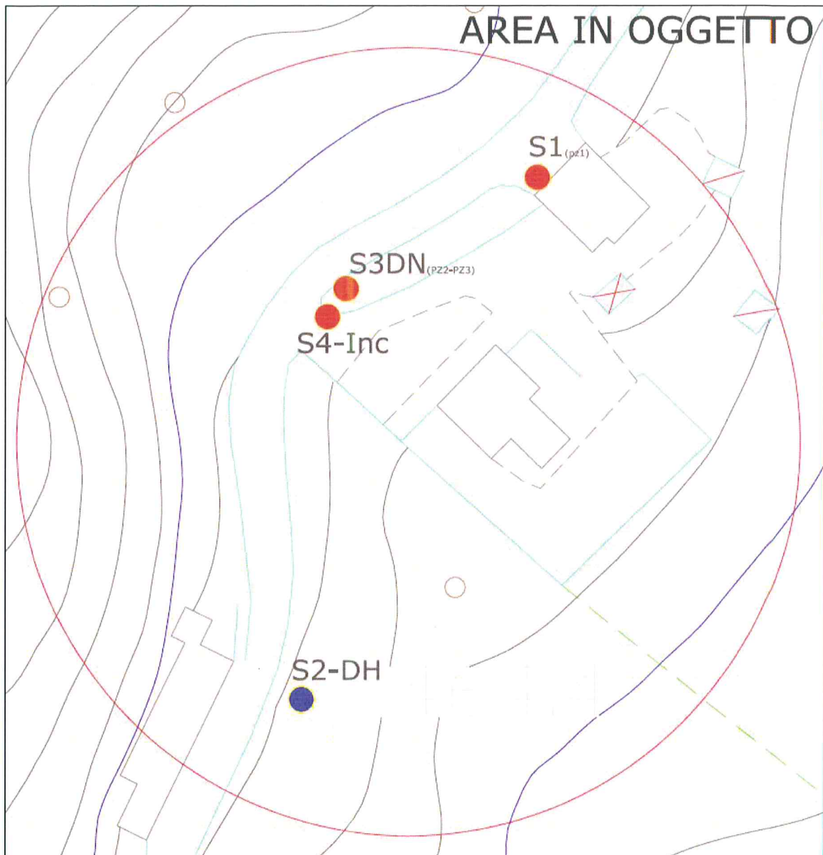
Figura 4 – Planimetria con ubicazione delle verticali di indagine
