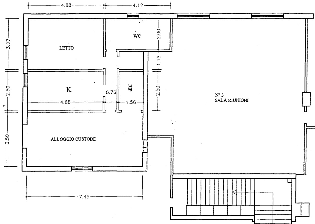
PIANTA ALLOGGIO CUSTODE PALATEDESCHI 1:100
